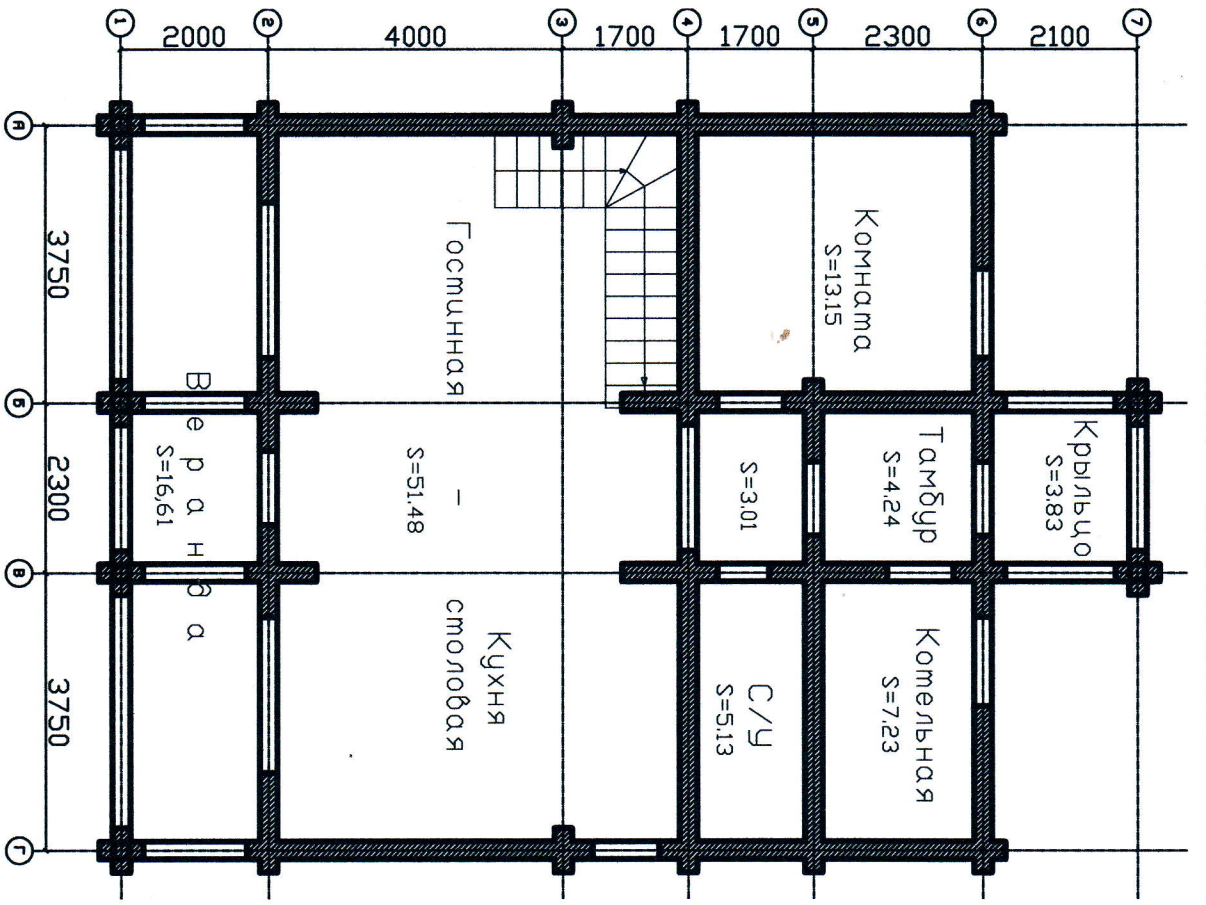
План 1этаж
