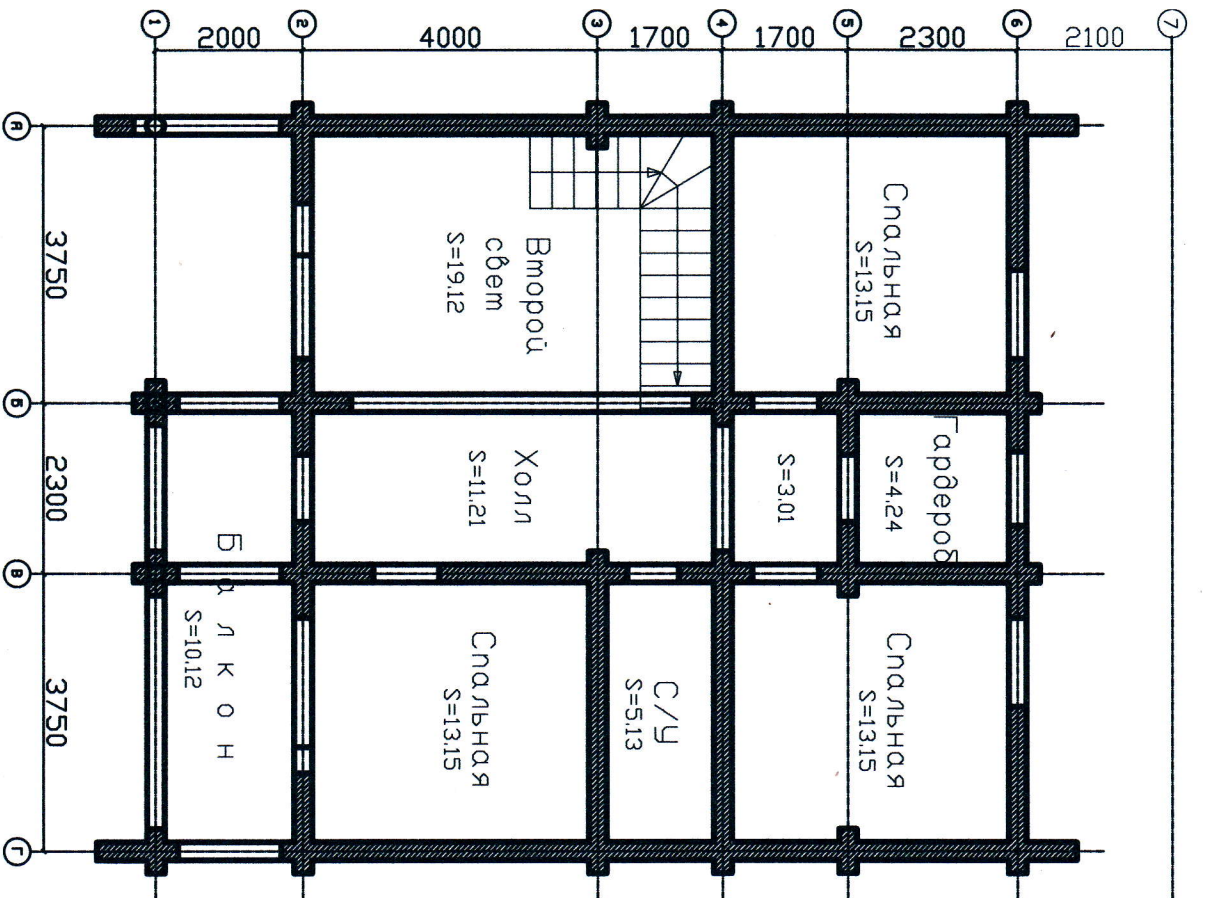
План 2этаж
